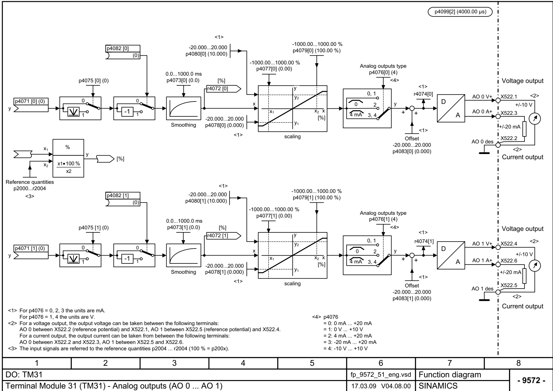
Fig. 3-372 9572 – Analog outputs (AO 0 ... AO 1)
