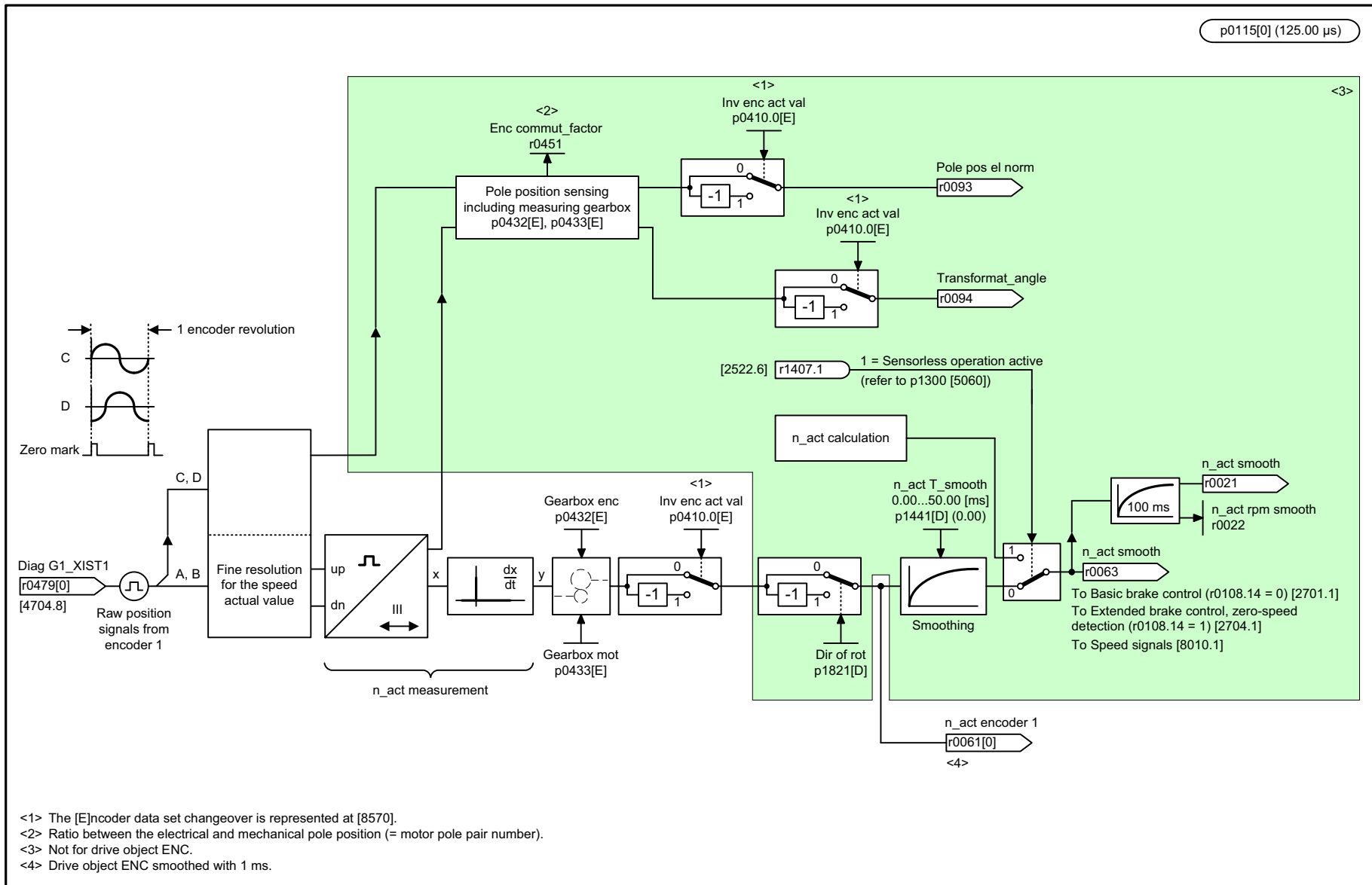
Fig. 3-185 4710 – Speed actual value and pole position sensing, encoder 1
