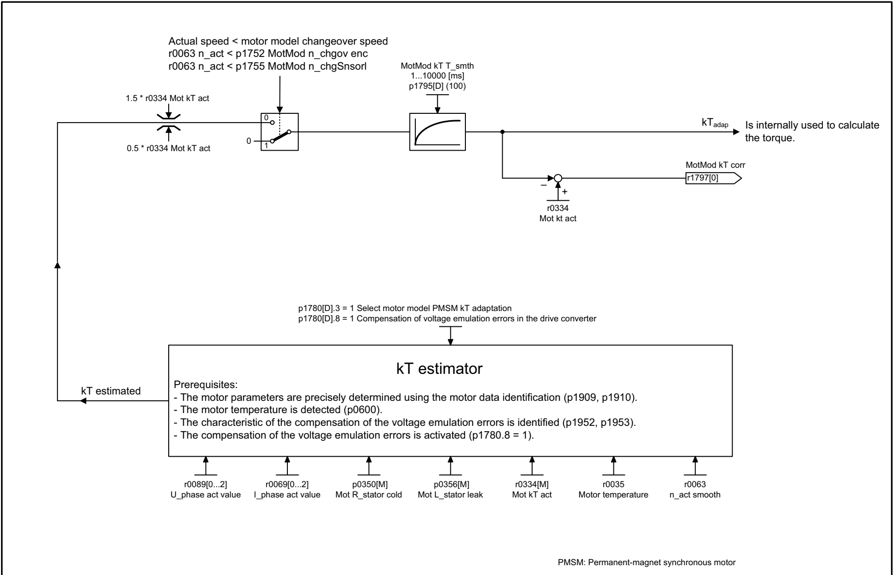
Fig. 3-262 7008 – kT estimator
