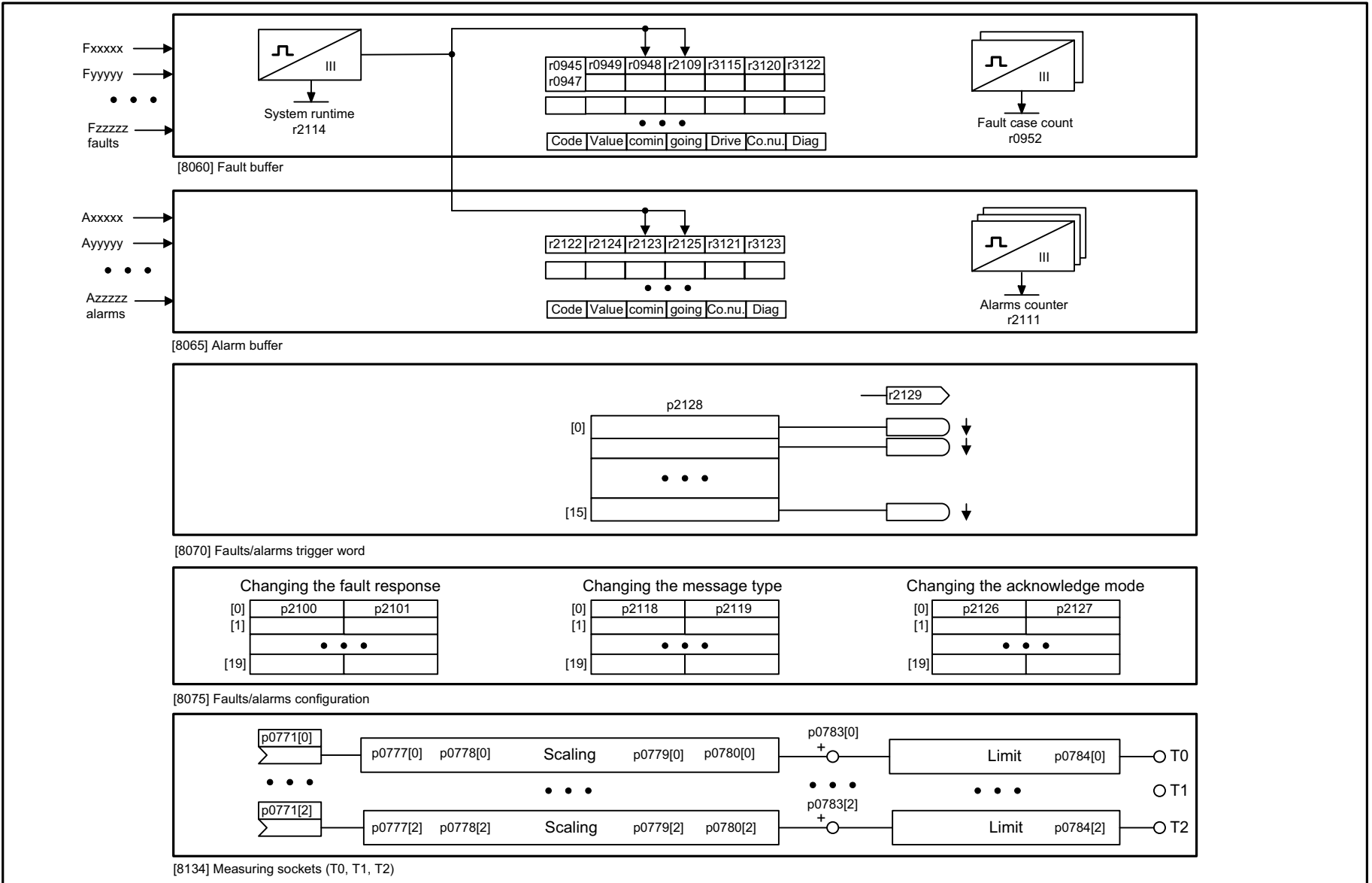
Fig. 3-304 8050 – Overview
