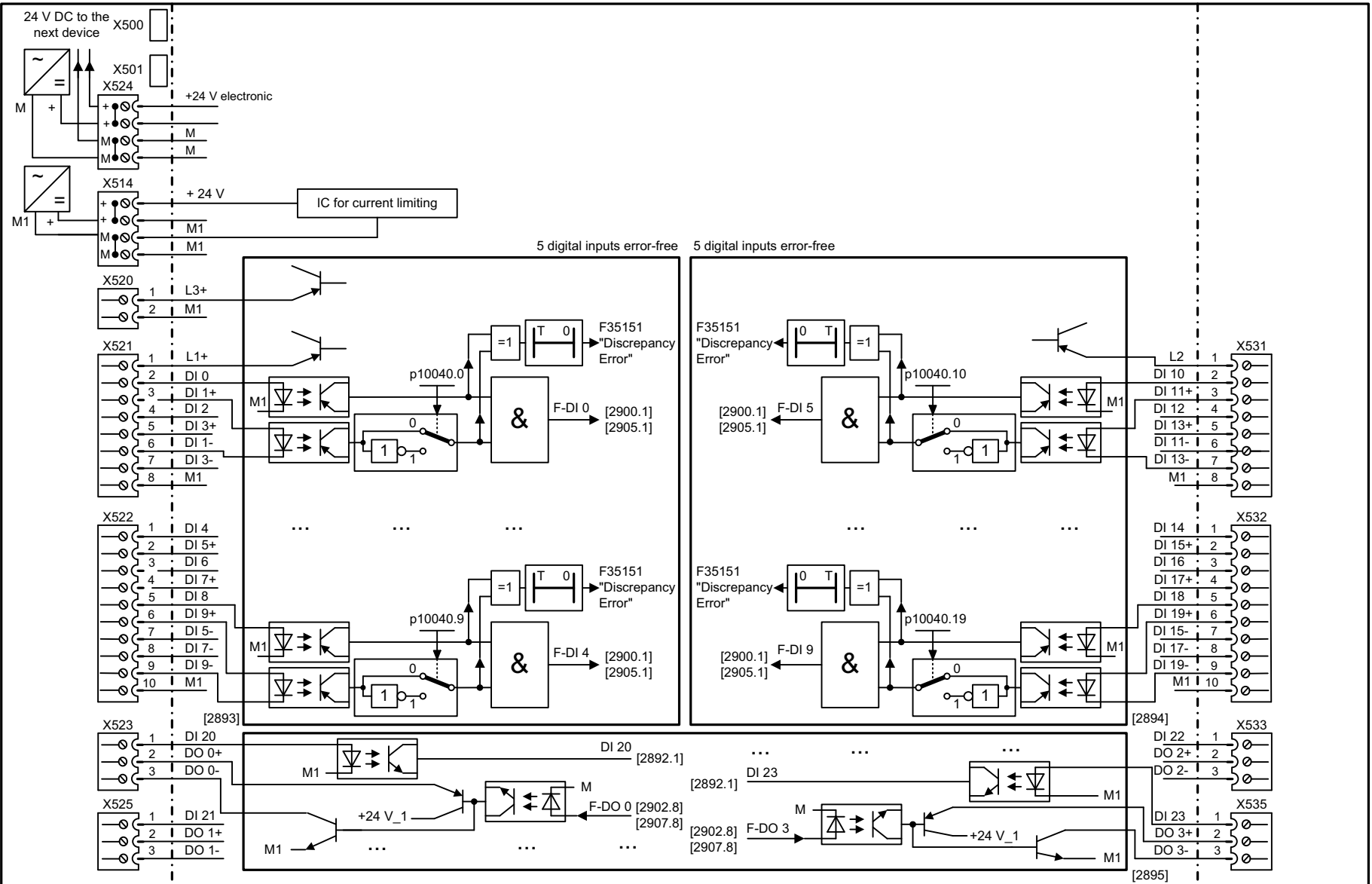
Fig. 3-137 2890 – Overview
