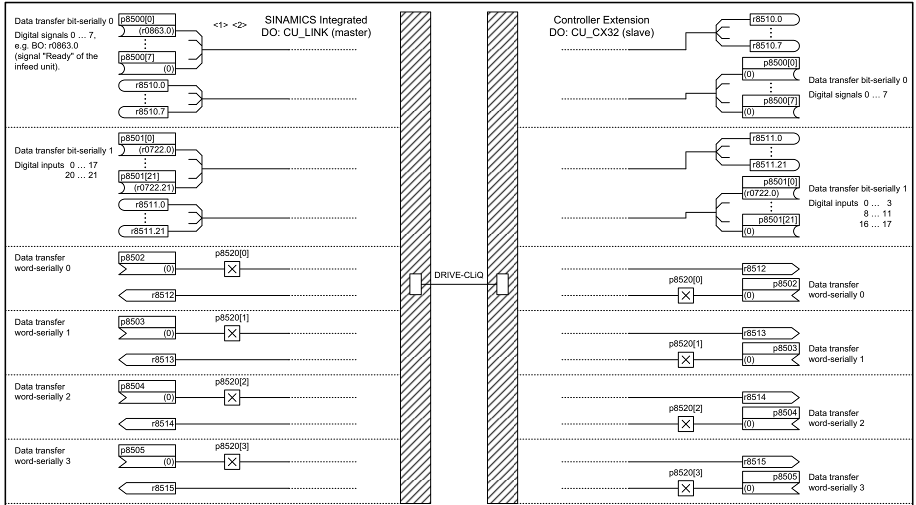
Fig. 3-25 2194 – CU_CX32/CU_LINK
