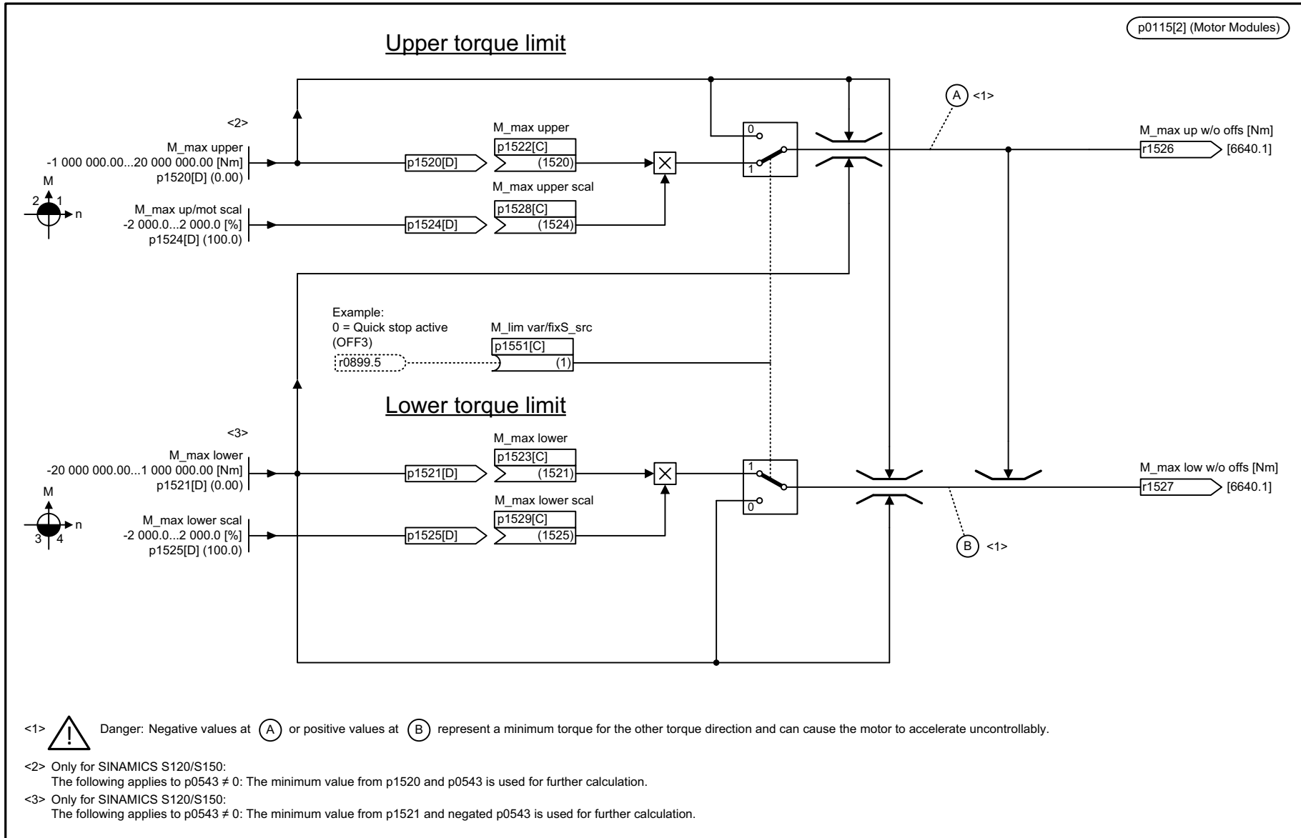
Fig. 3-242 6630 – Upper/lower torque limit
