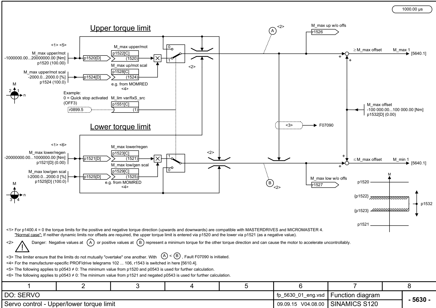
Fig. 3-218 5630 – Upper/lower torque limit
