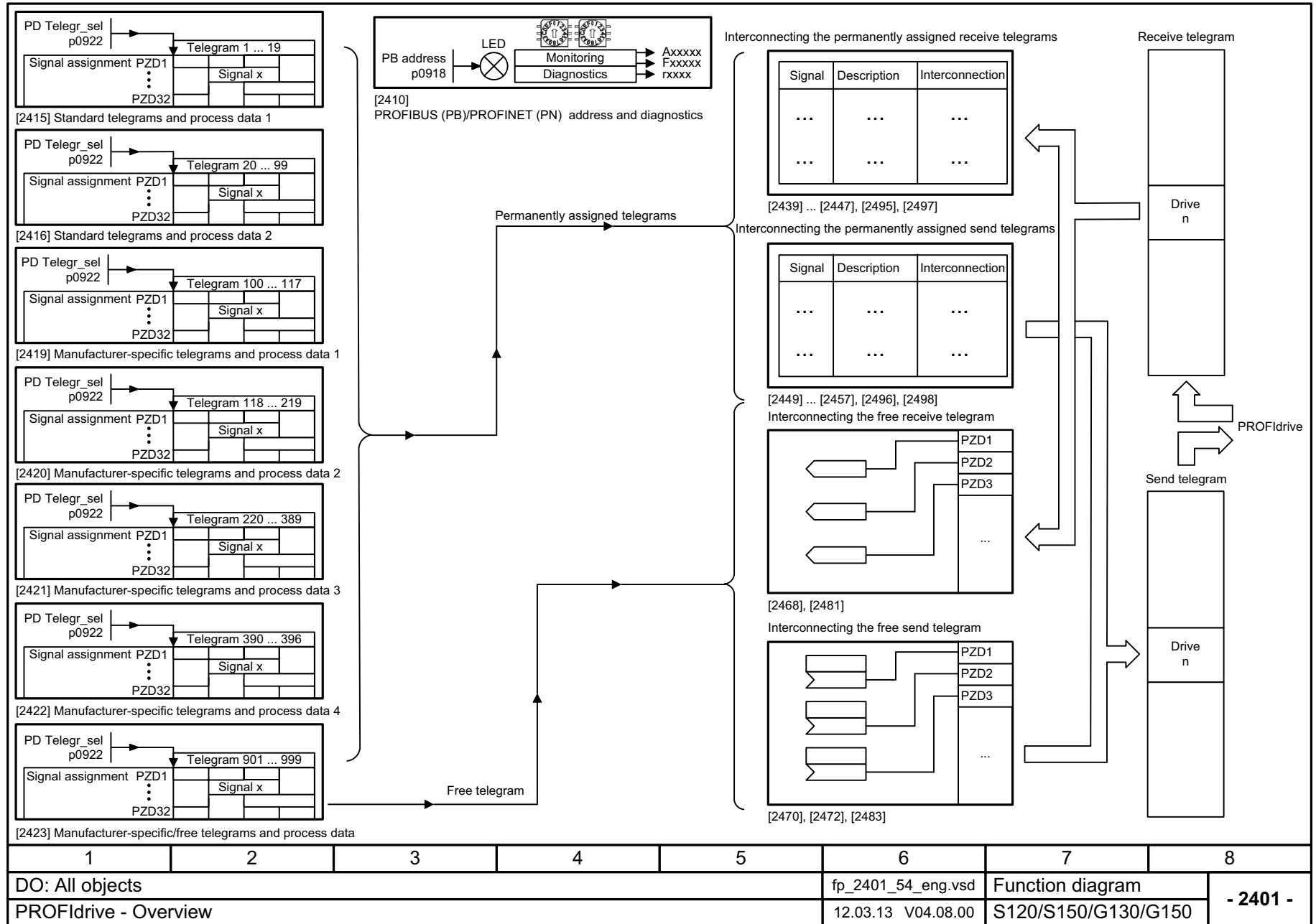
Fig. 3-34 2401 – Overview
