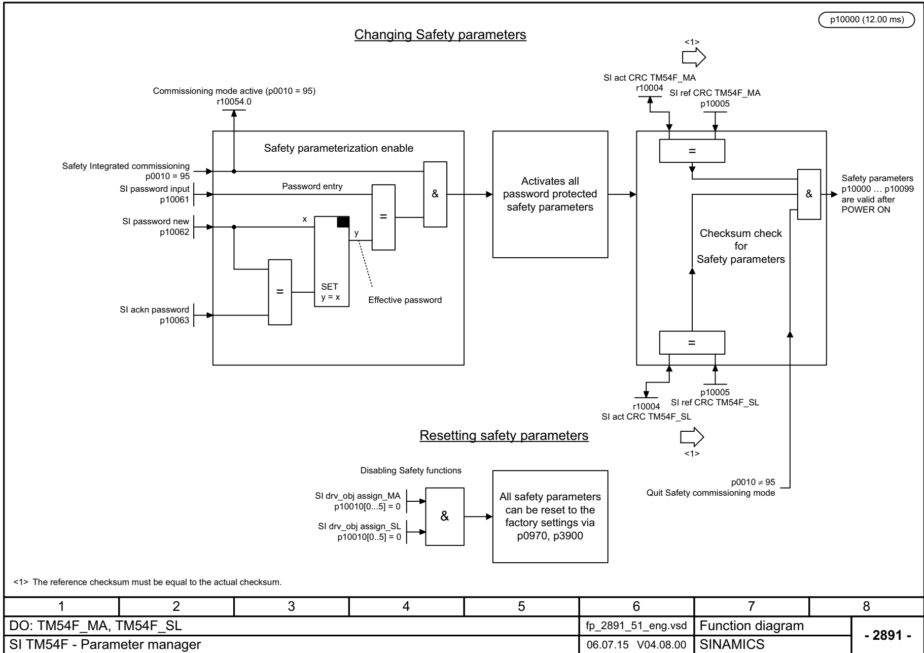
Fig. 3-138 2891 – Parameter manager
