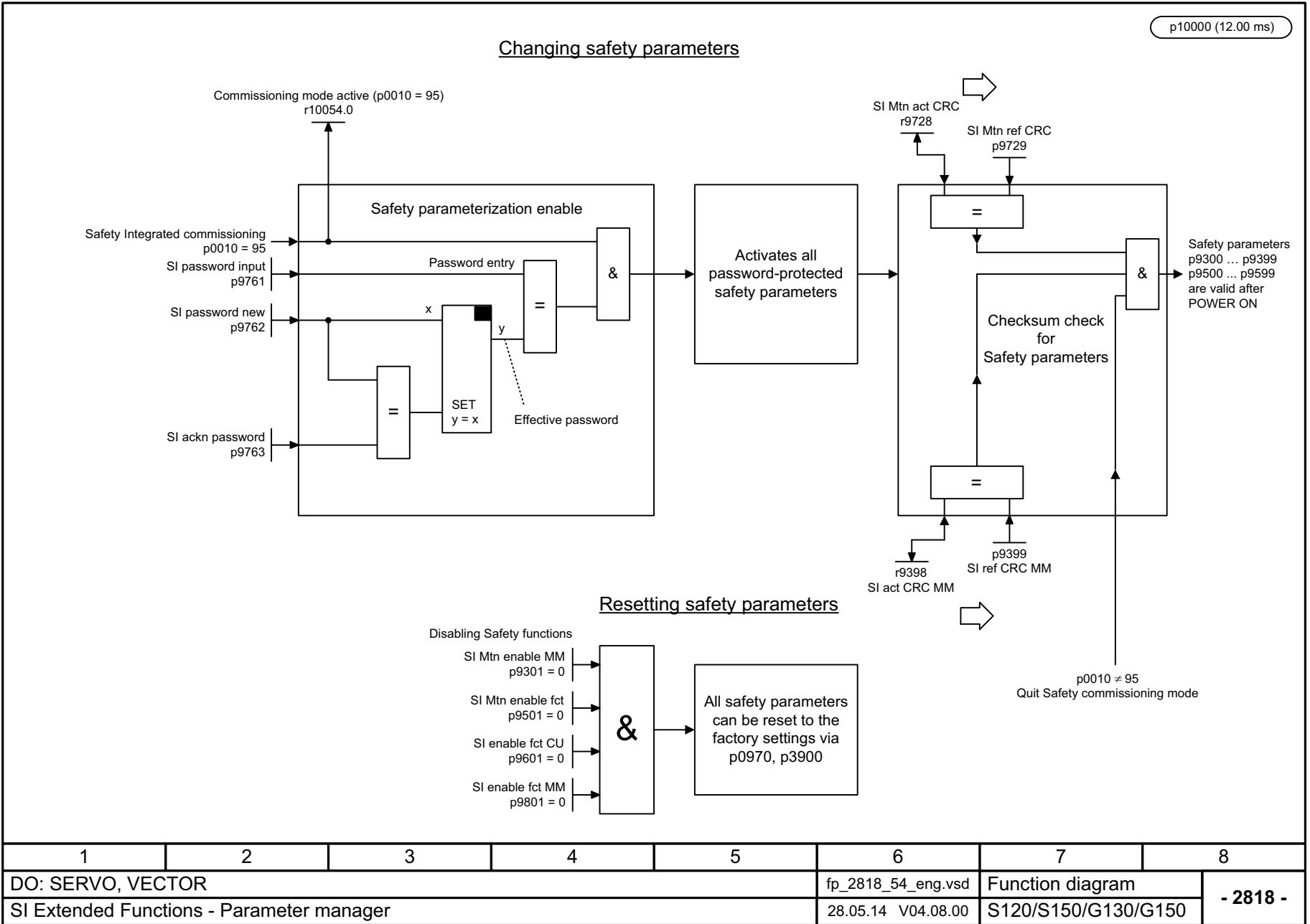
Fig. 3-118 2818 – Parameter manager
