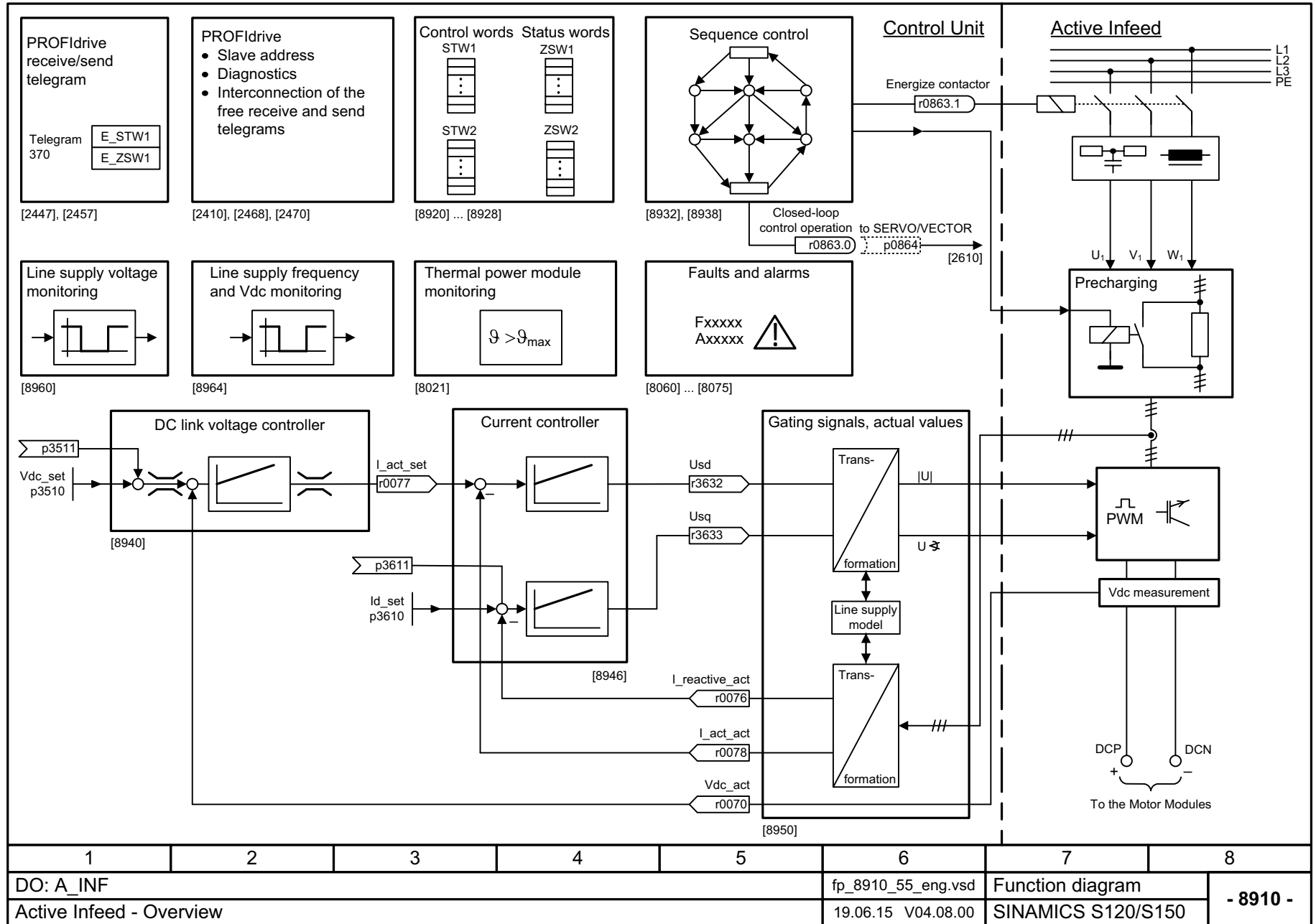
Fig. 3-333 8910 – Overview
