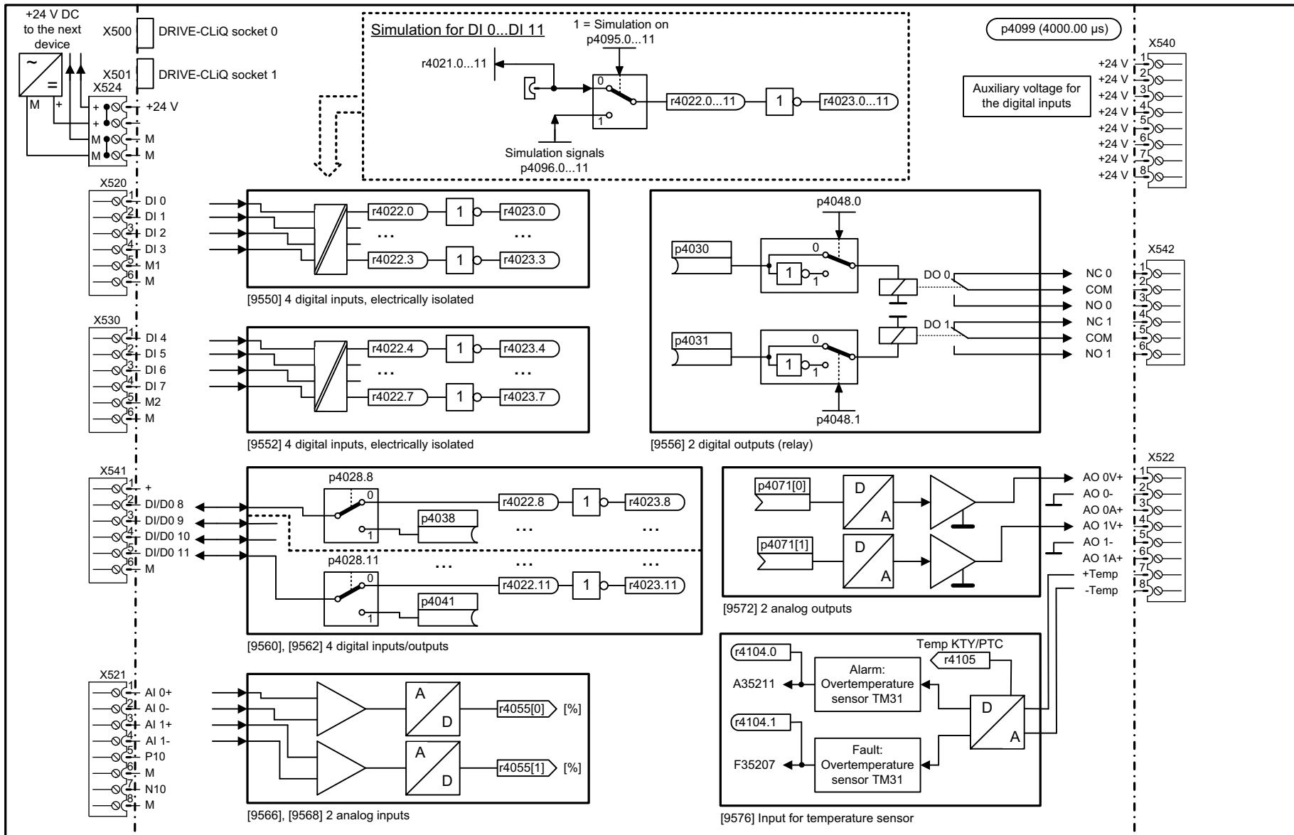
Fig. 3-364 9549 – Overview
