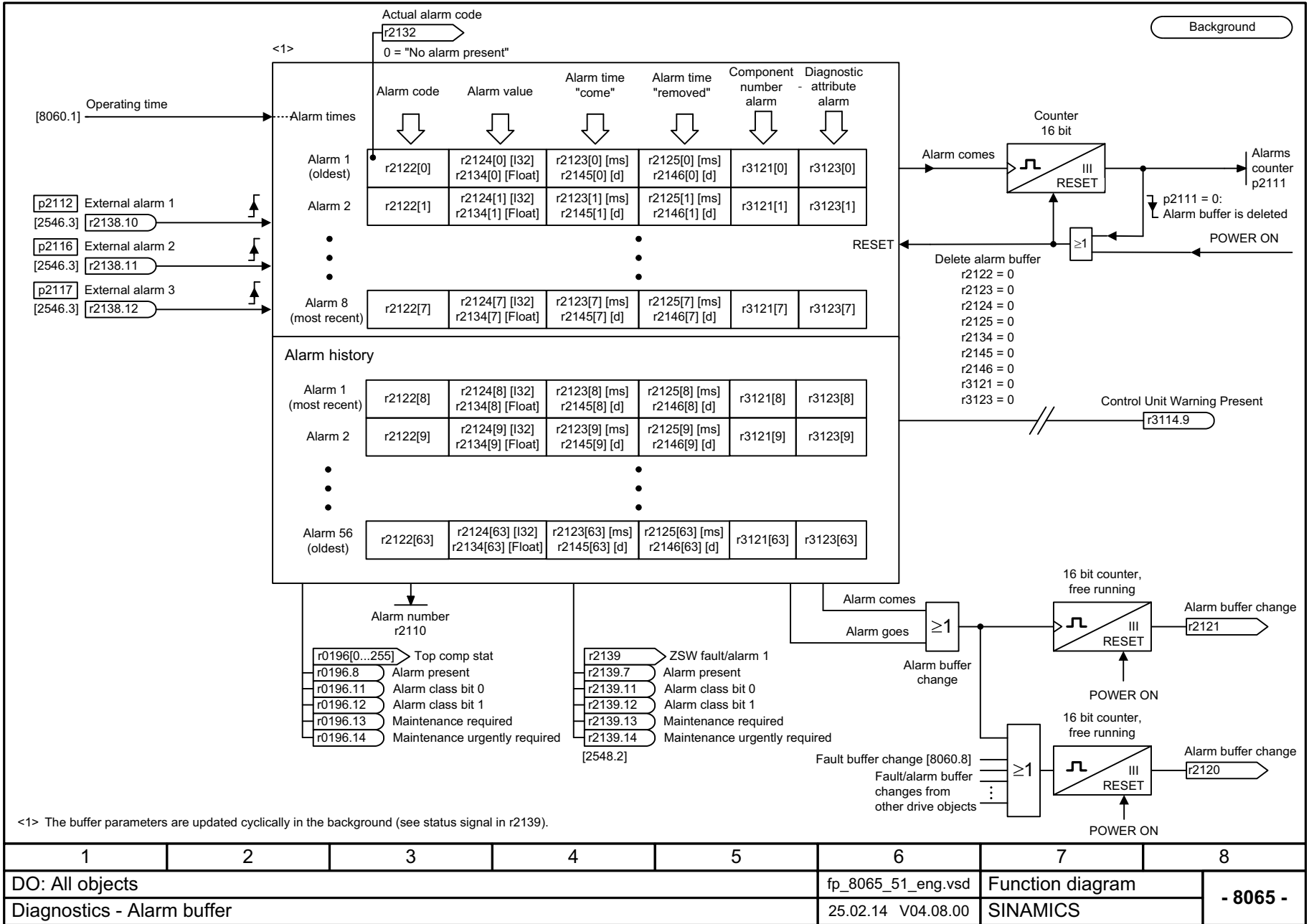
Fig. 3-306 8065 – Alarm buffer
