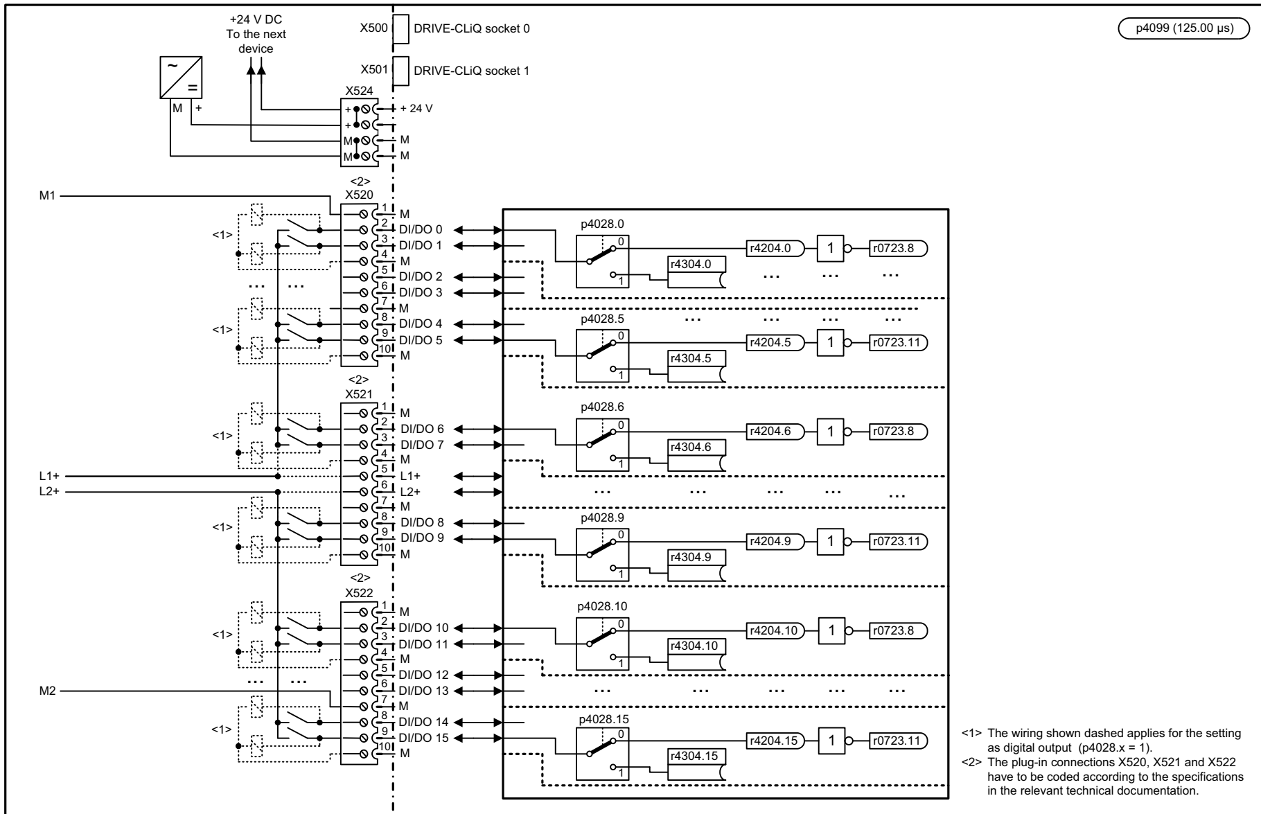
Fig. 3-363 9419 – Overview
