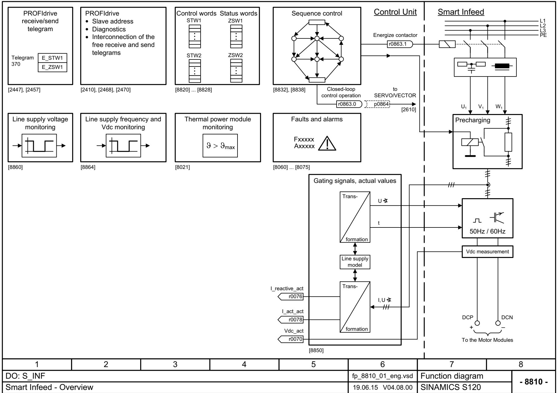
Fig. 3-324 8810 – Overview
