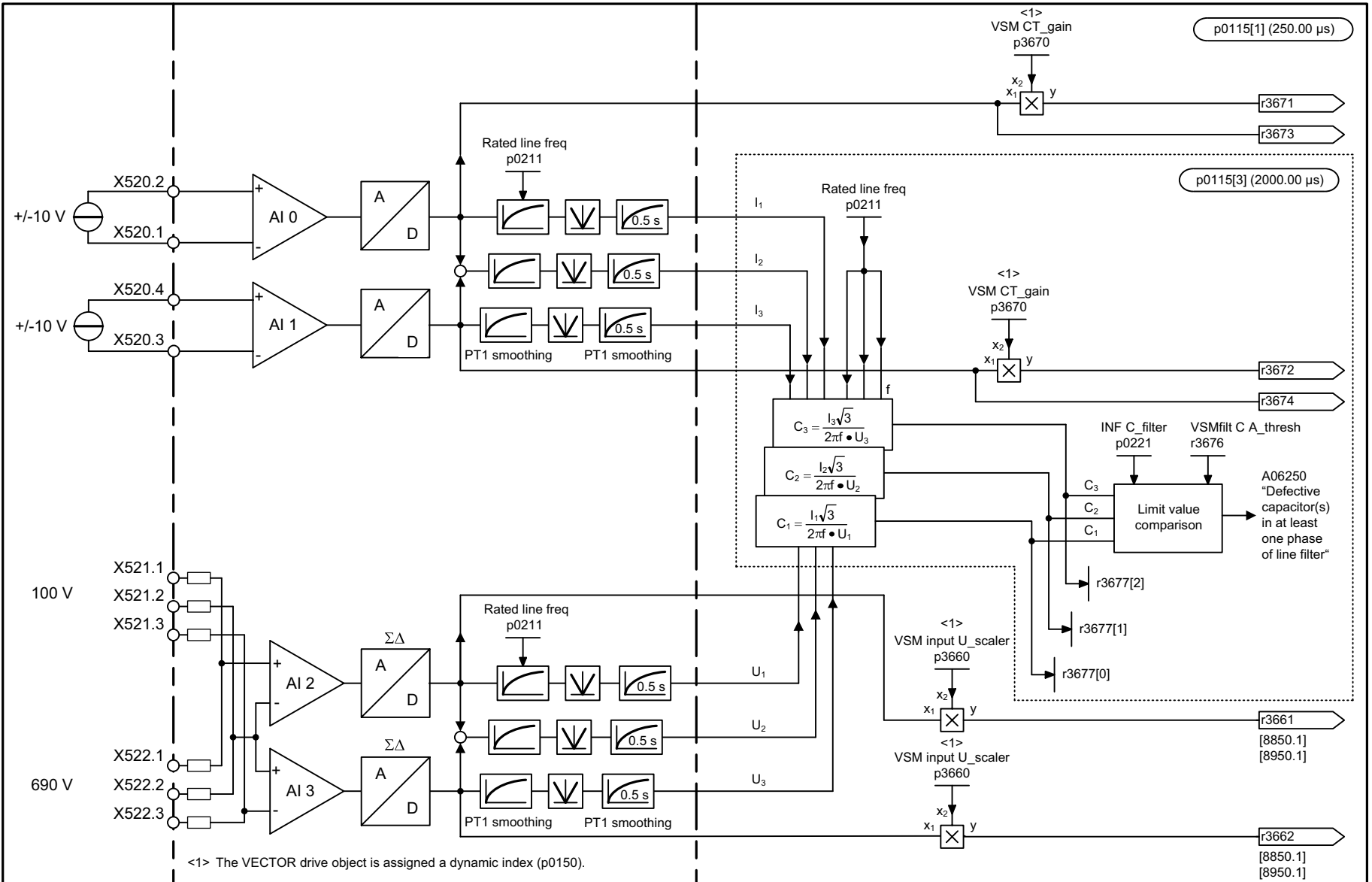
Fig. 3-396 9880 – Analog inputs (AI 0 ... AI 3)
