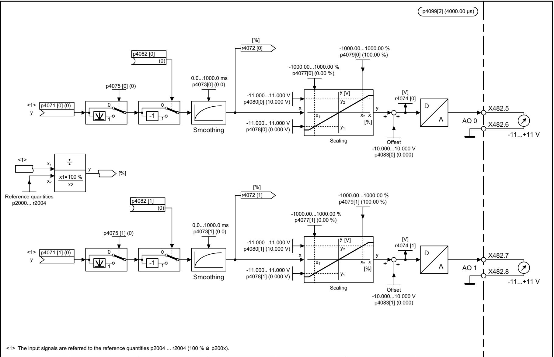
Fig. 3-351 9106 – Analog outputs (AO 0 ... AO 1)
