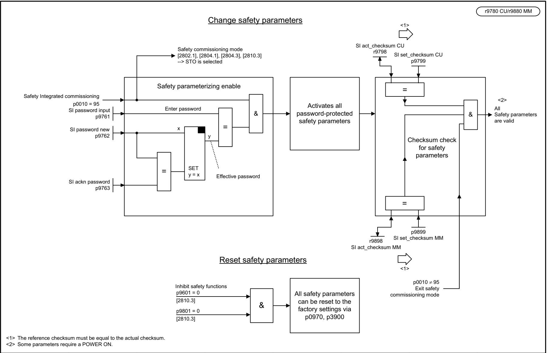
Fig. 3-111 2800 – Parameter manager
