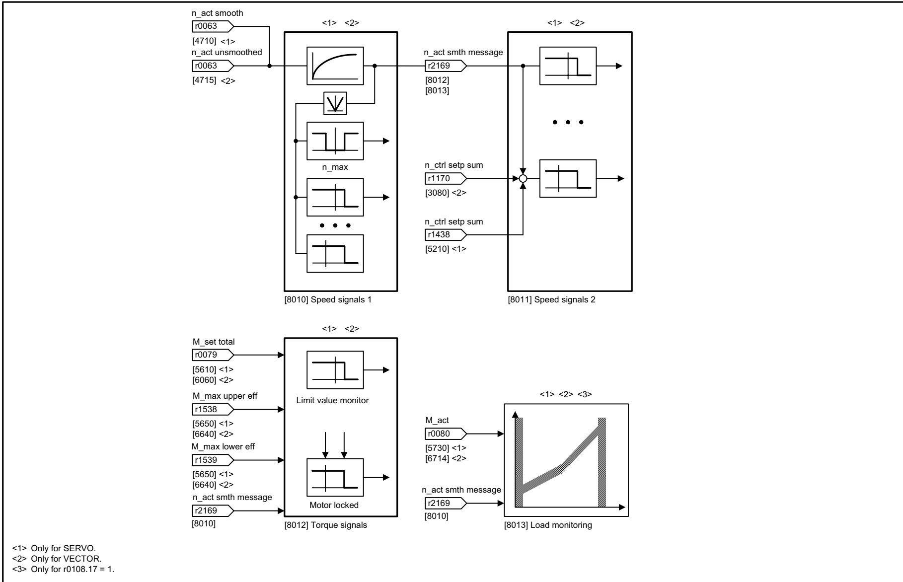
Fig. 3-292 8005 – Overview
